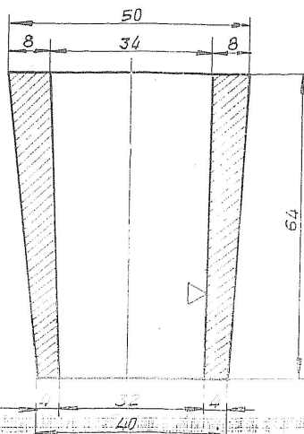
A-A KESİTİ
